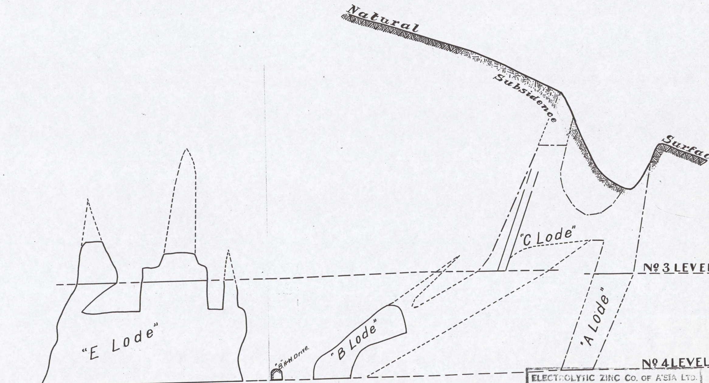
Nº9 SECTION
