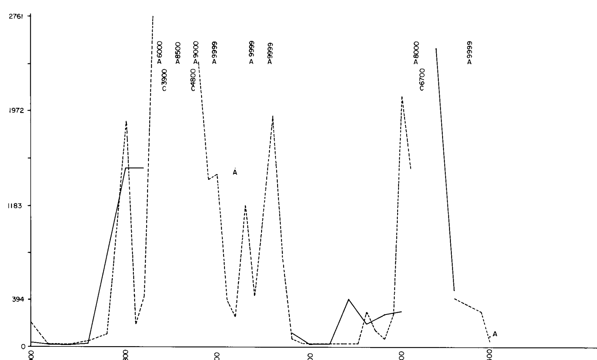
MANGANESE
