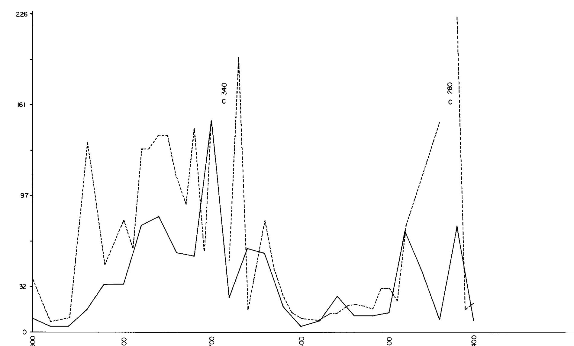
ZINC
